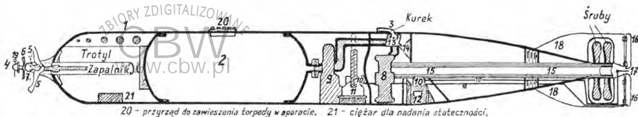
20 - przyrząd do zawieszania torpedy w aparacie. 21 - ciężar dla nadania stateczności.
