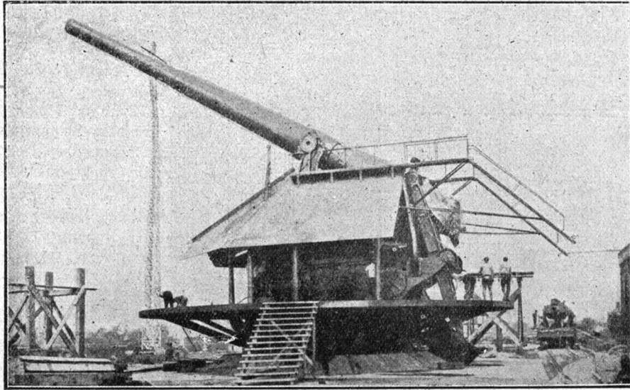
16 calowe (40 cm) działo amerykańskie na podstawie znikającej, wzoru 1919 Największy kąt podniesienia 30°, najmniejszy—5°, szybkość wylotowa 900 m/sek., waga pocisku 1.200 kg, największa donośność 34.500 m.
