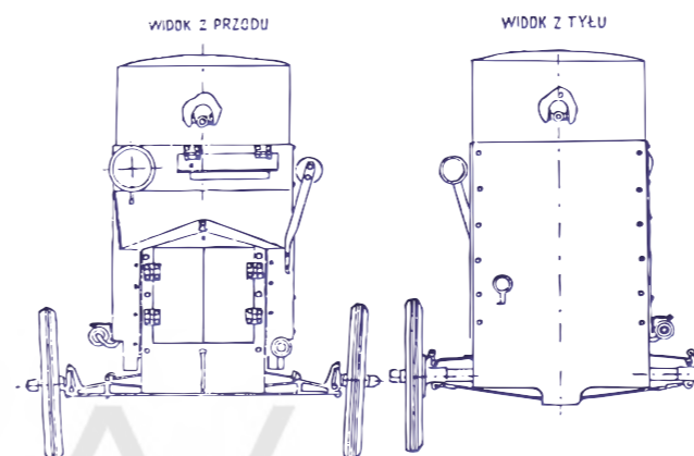
Projekt samochodu pancernego Ford FT-B mod. 1920 (II seria) konstrukcji inż. Tadeusza Tańskiego.
