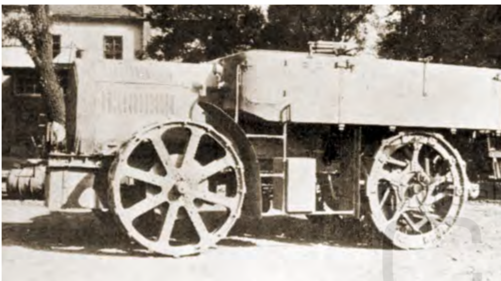
Ciągnik artyleryjski MZW M 17 Austro-Daimler (4x4). MZW M17 Austro-Daimler (4x4) artillery tractor.
