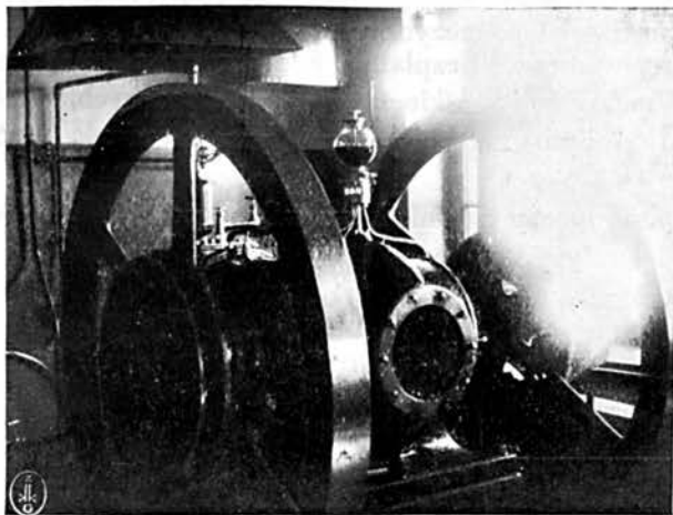
Motor „Perkun” uruchamiający elektrownię pułkową.
