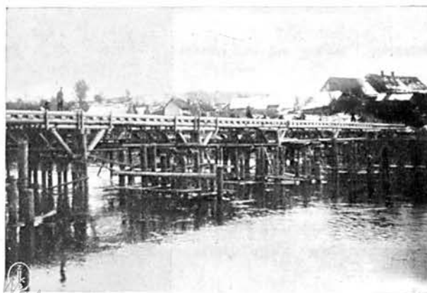
Budowa stałego mostu szosowego 20-tonnowego na rzece Pilicy pod Inowłodziem w roku 1926-ym. Buduje 13 Baon Saperów.
