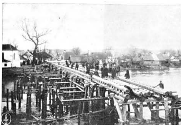
Budowa stałego mostu szosowego 20-tonnowego na rzece Pilicy pod Inowłodziem w roku 1926-ym. Buduje 13 Baon Saperów.
