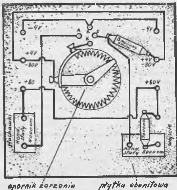
Rys. 2. Schemat połączeń.
