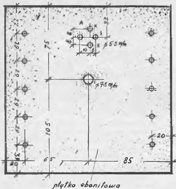
Rys. 1. Rozmieszczenie otworów na płytce.
